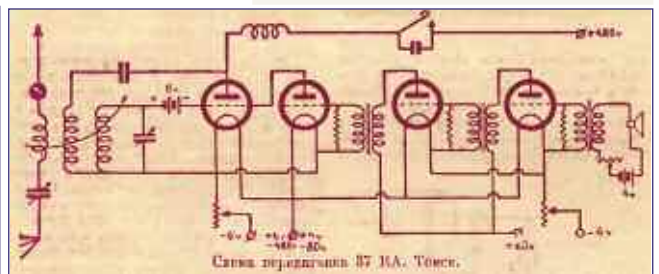
Схема передатчика 37RA.
